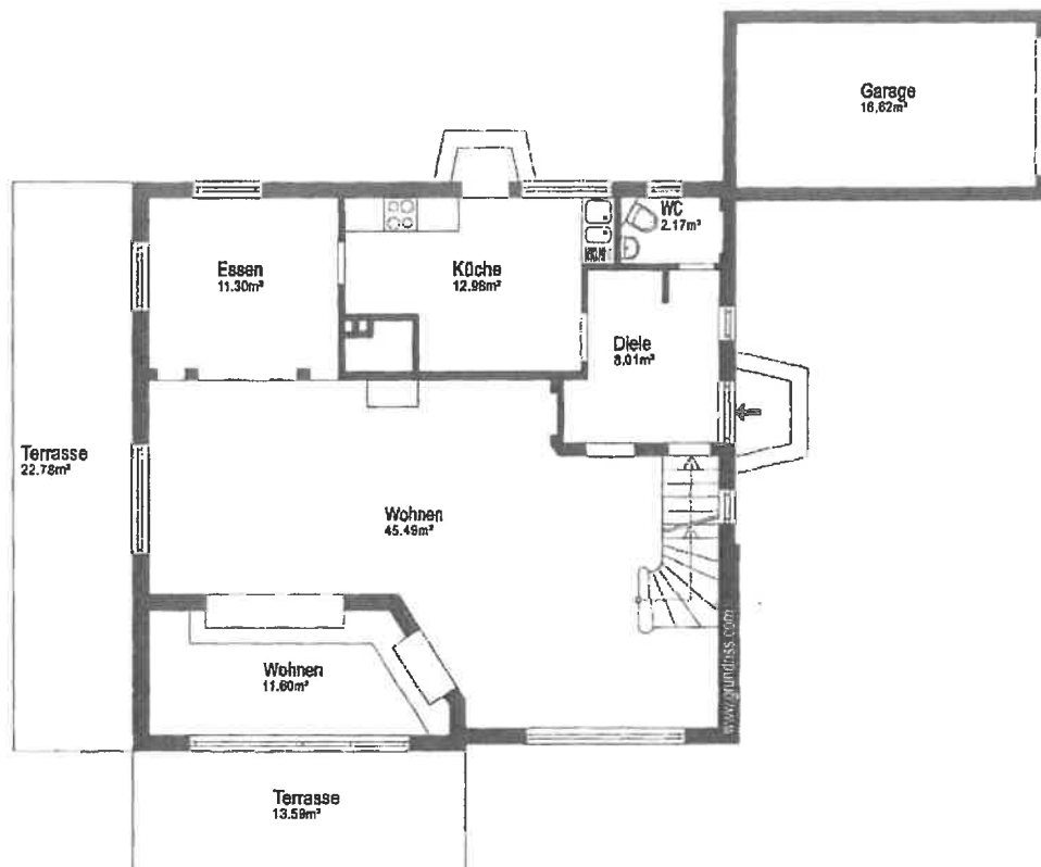
Erdgeschoss
